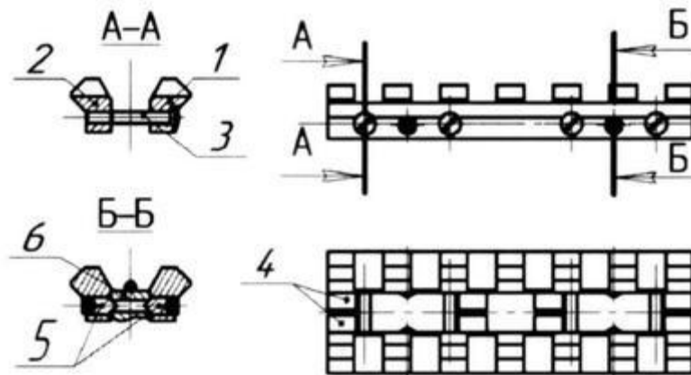
Рисунок 1. Кронштейн Weaver на ИЖ-27 ЭТМИ.734348.019
