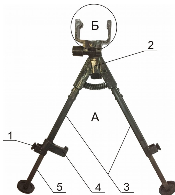
1- удлинитель опоры; 2 – основание; 3 – опора; 4 – защелка; 5 – фиксатор А – опорная часть; Б – узел крепления к оружию
