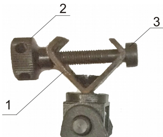
1 – «щеки»; 2 – гайка; 3 – крепежный винт
